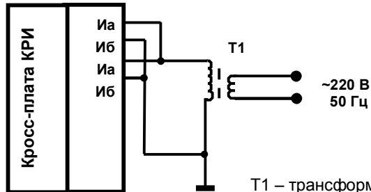
Рисунок 1.15 – Схема проверки импульсных входов
